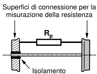
Fig. 1 Rappresentazione schematica della sala montata con isolamento elettrico, resistenza di ponte e superfici di misura.
